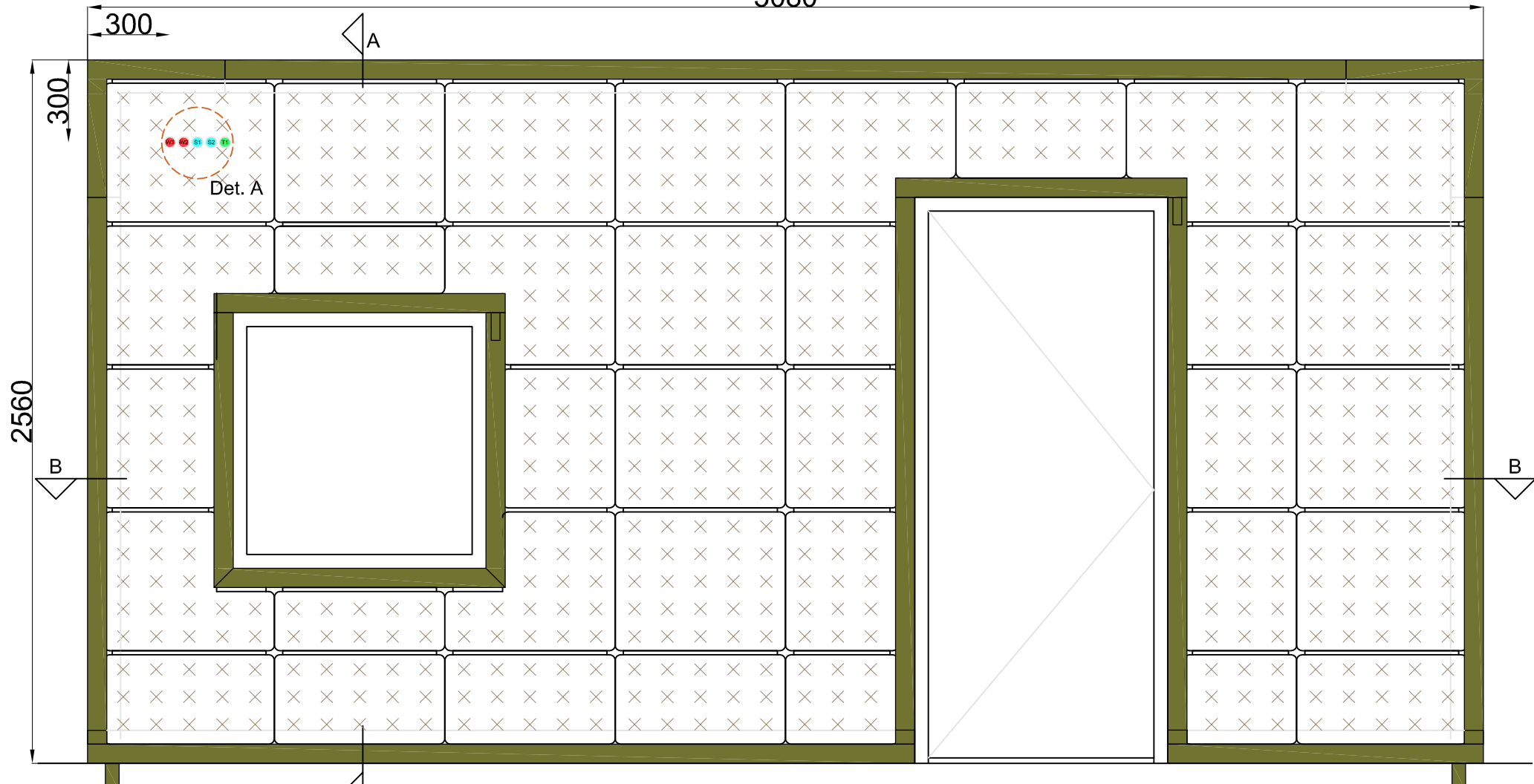
Vorderansicht
