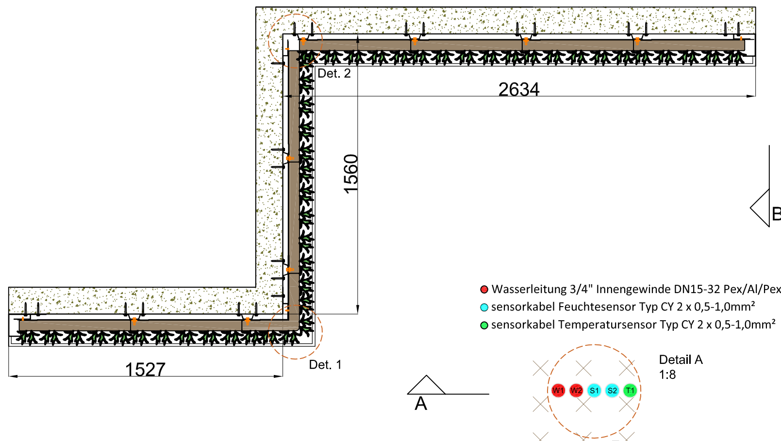
Ansicht A.
