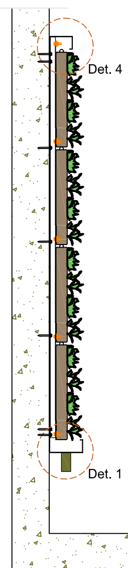
Querschnitt A-A
