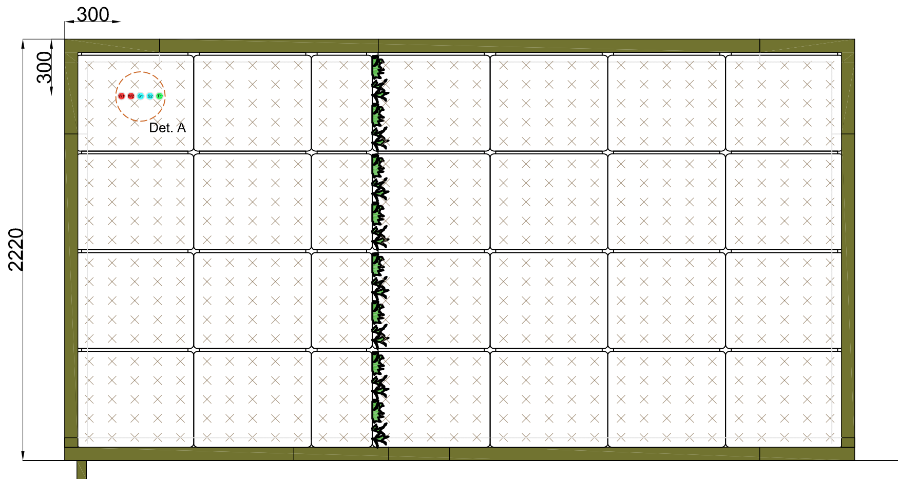
Ansicht A.
