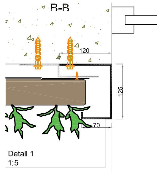
Querschnitt
