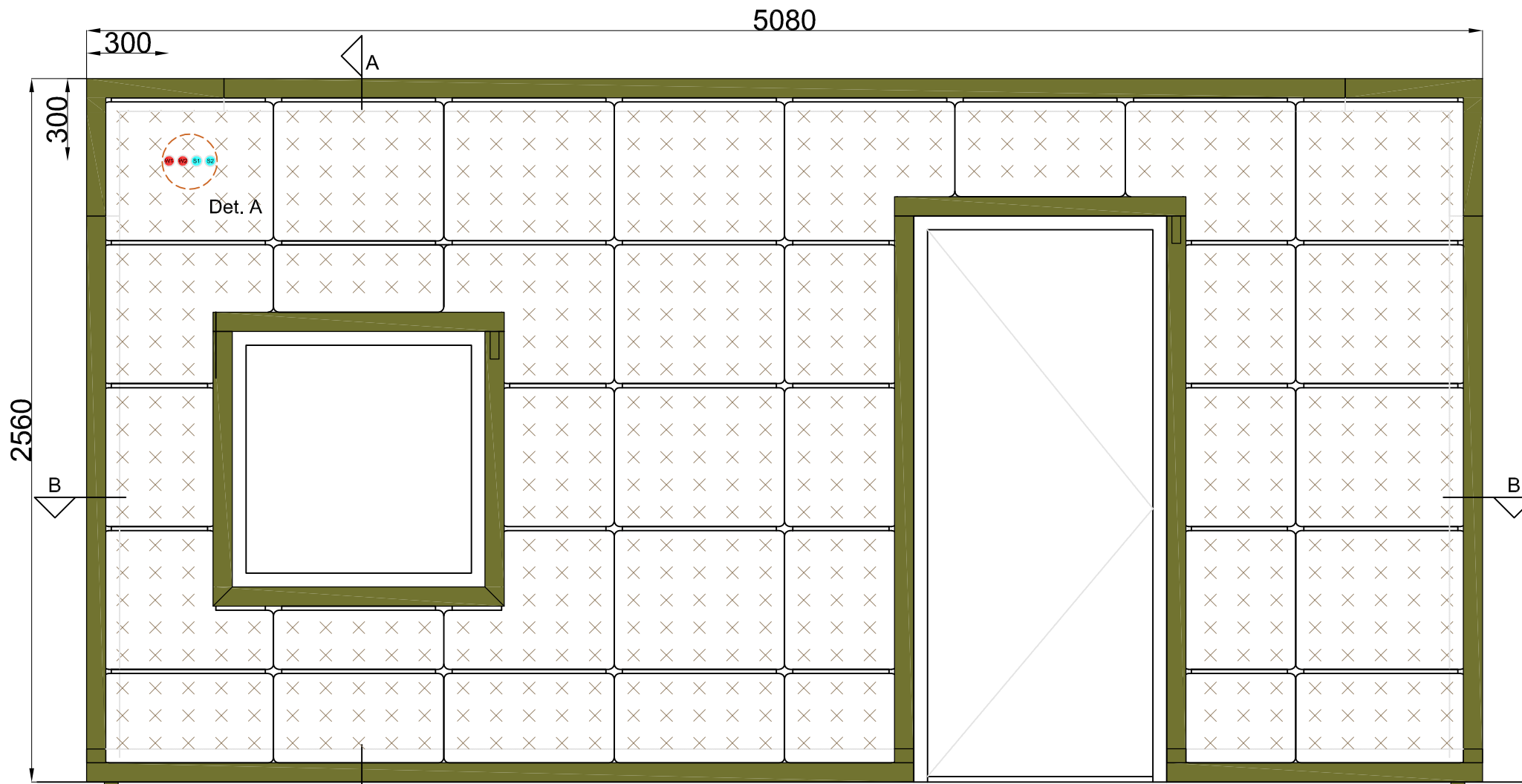
Vorderansicht
