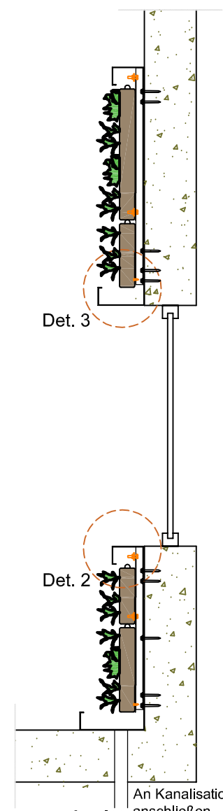
Querschnitt A-A
