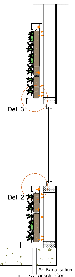
Querschnitt A-A
