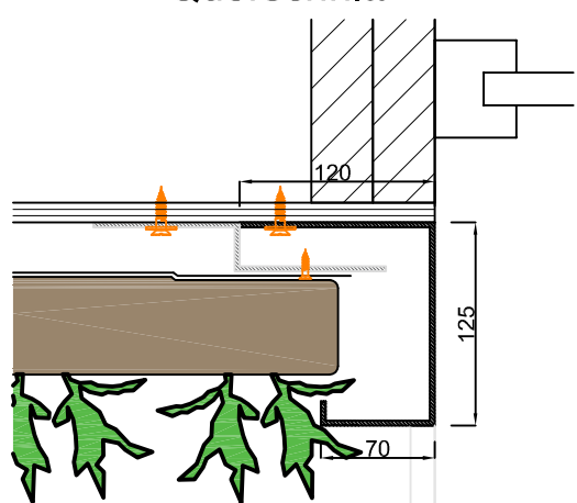
Querschnitt
