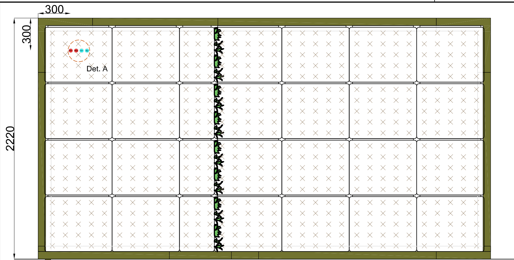
Ansicht A.
