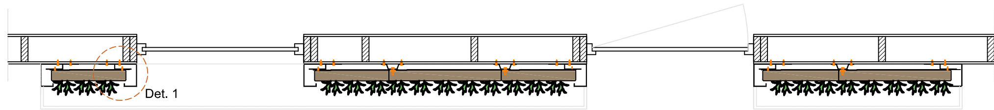
Querschnitt
