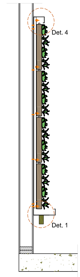
Querschnitt A-A
