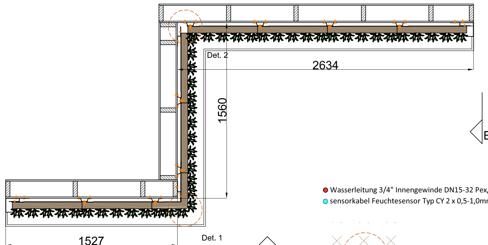
Ansicht A.
